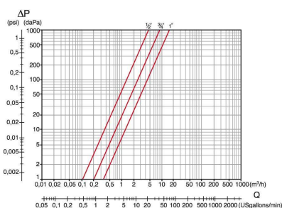
LoadLossChart
