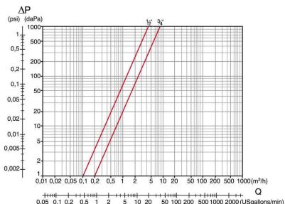
LoadLossChart
